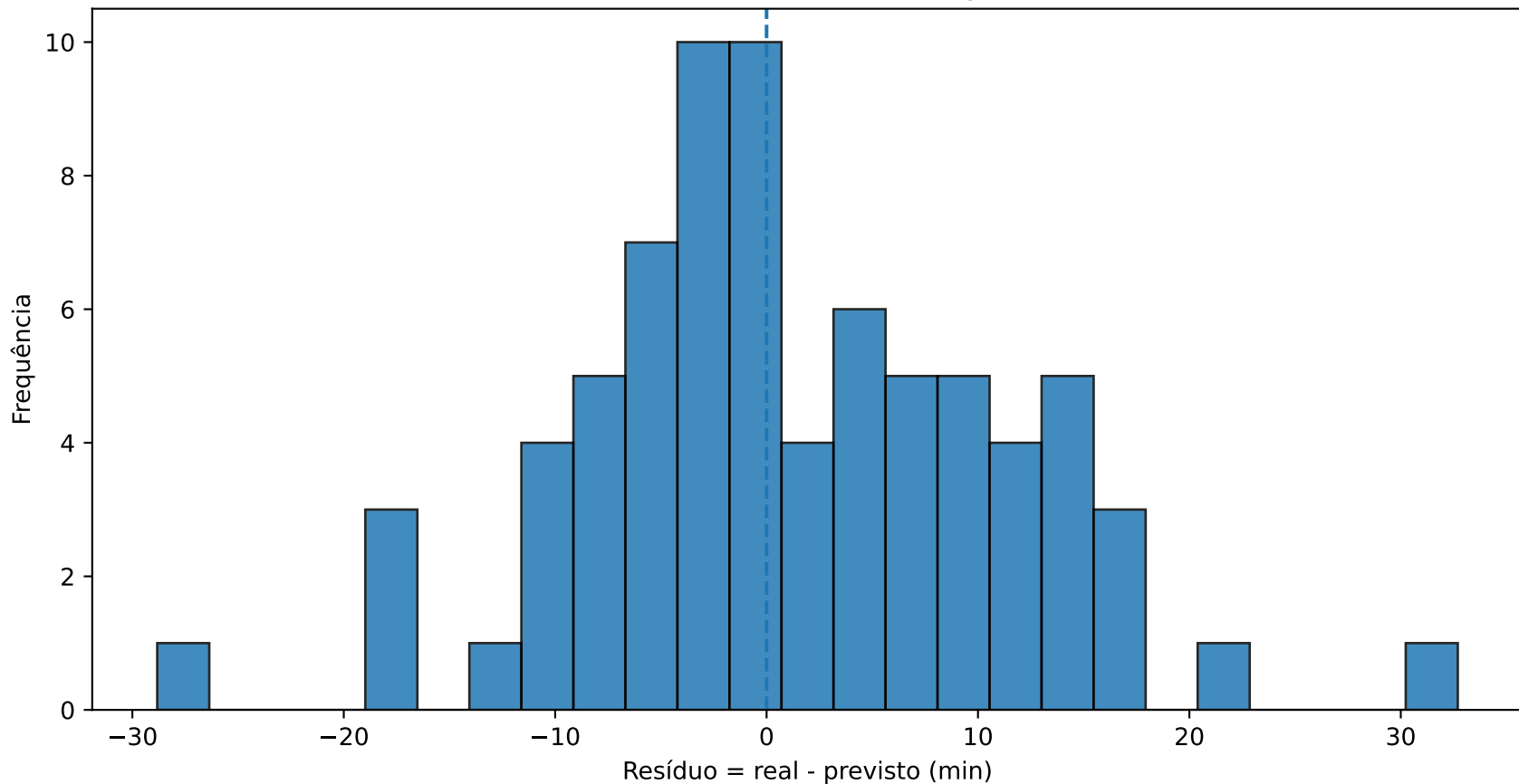
Distribuição dos resíduos - PyTorch
